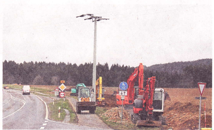
Vier Bagger sind neben der B85 bei Linden schon seit Dienstag am Werk. Hier entsteht zunächst ein Schmutzwasserkanal.
